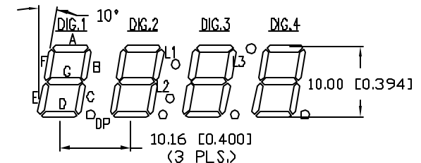
DIGIT DETAIL
