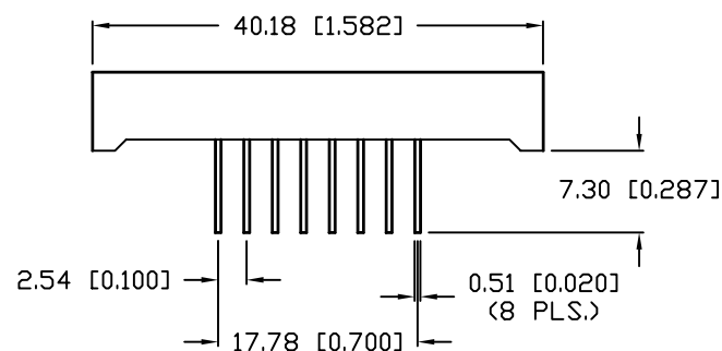
DIGIT DETAIL
