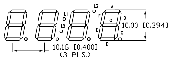
DIGIT DETAIL
