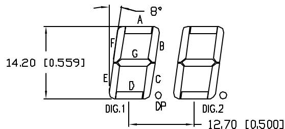
DIGIT DETAIL
