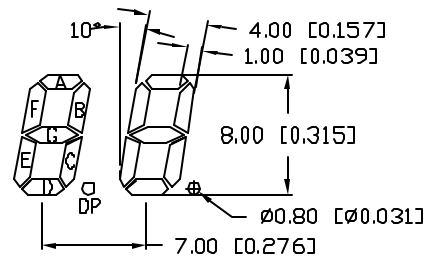
DIGIT DETAIL
