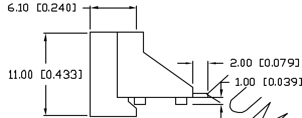
DIGIT DETAIL
