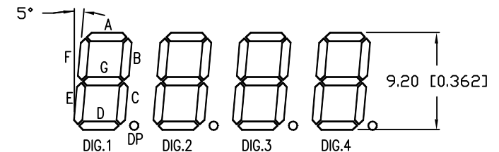
DIGIT DETAIL
