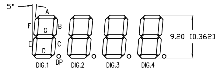
DIGIT DETAIL
