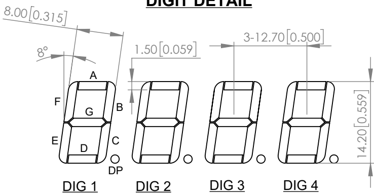
DIGIT DETAIL
