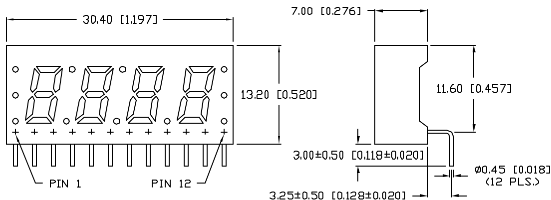
DIGIT DETAIL
