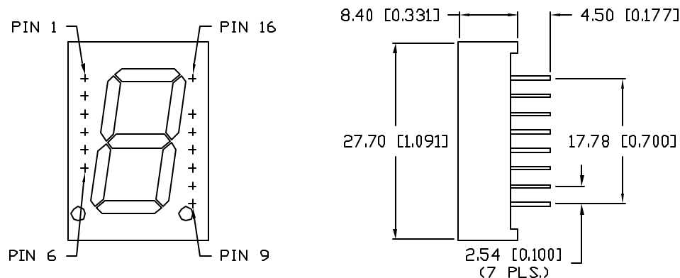
DIGIT DETAIL
