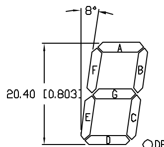
DIGIT DETAIL
