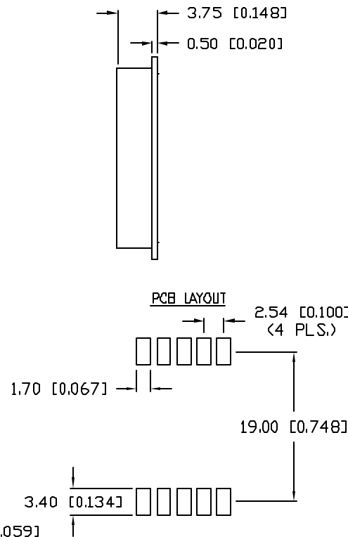
DIGIT DETAIL
