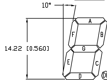
DIGIT DETAIL
