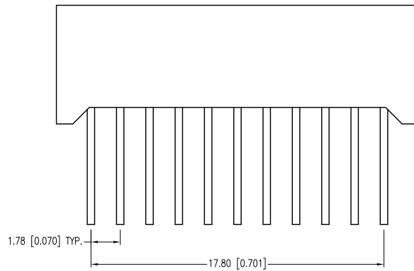
DIGIT DETAIL
