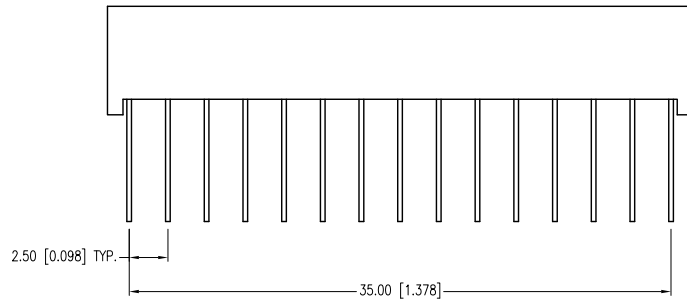
DIGIT DETAIL
