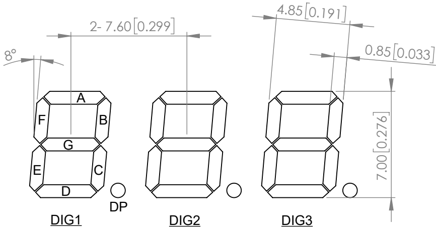
DIGIT DETAIL
