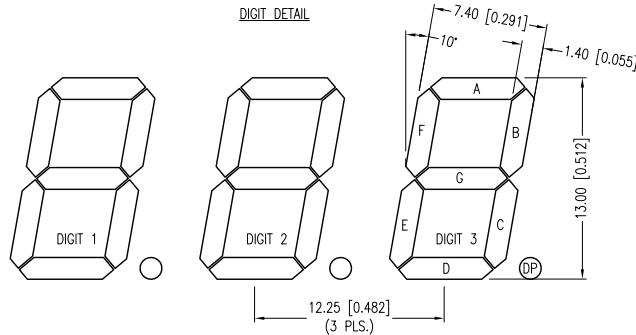
DIGIT DETAIL
