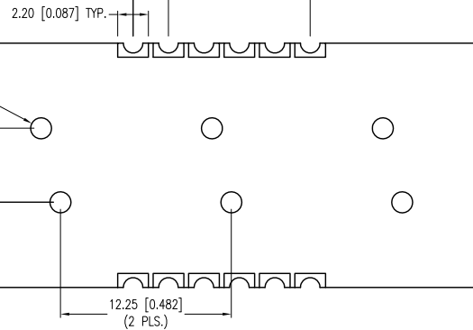
DIGIT DETAIL
