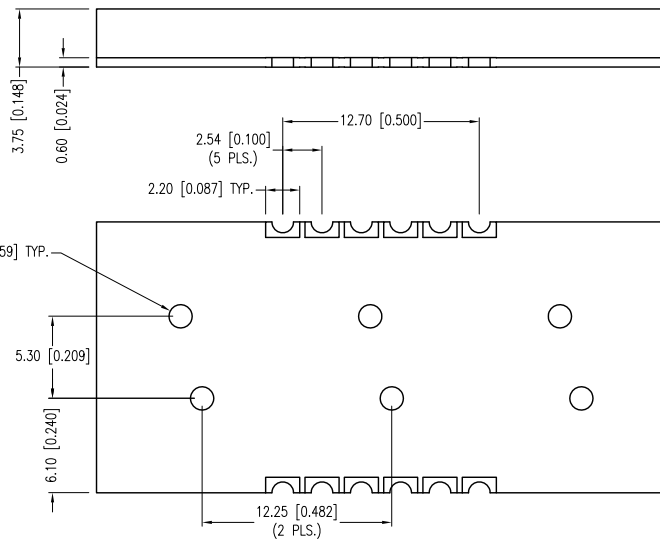
DIGIT DETAIL
